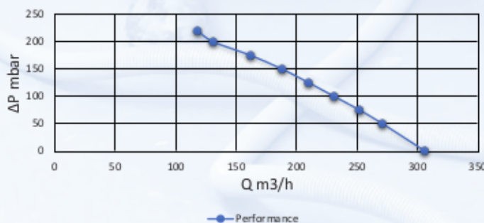
TKW22 2,2 kW
